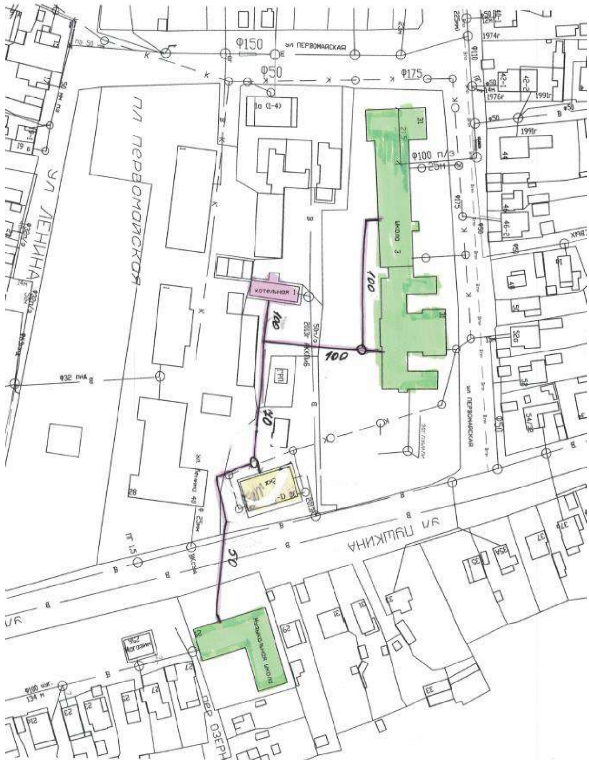
Рисунок 1.3.2.1 - Схема тепловых сетей котельной №1 г. Кинель
